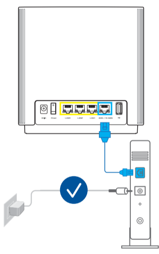
數據機後側
